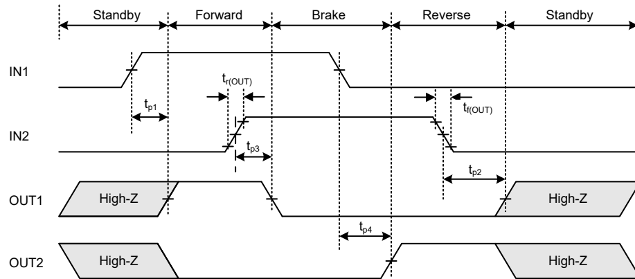
图 1. 活动周期的操作模式控制逻辑
