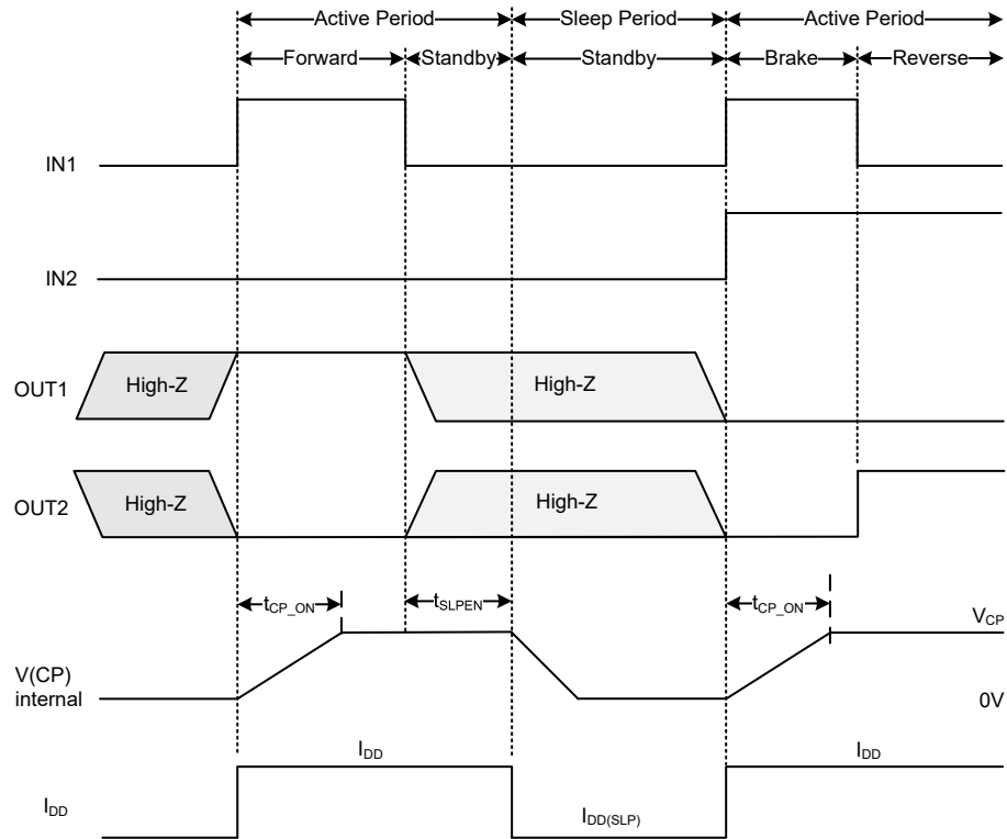
图 2. 操作模式控制时序图
