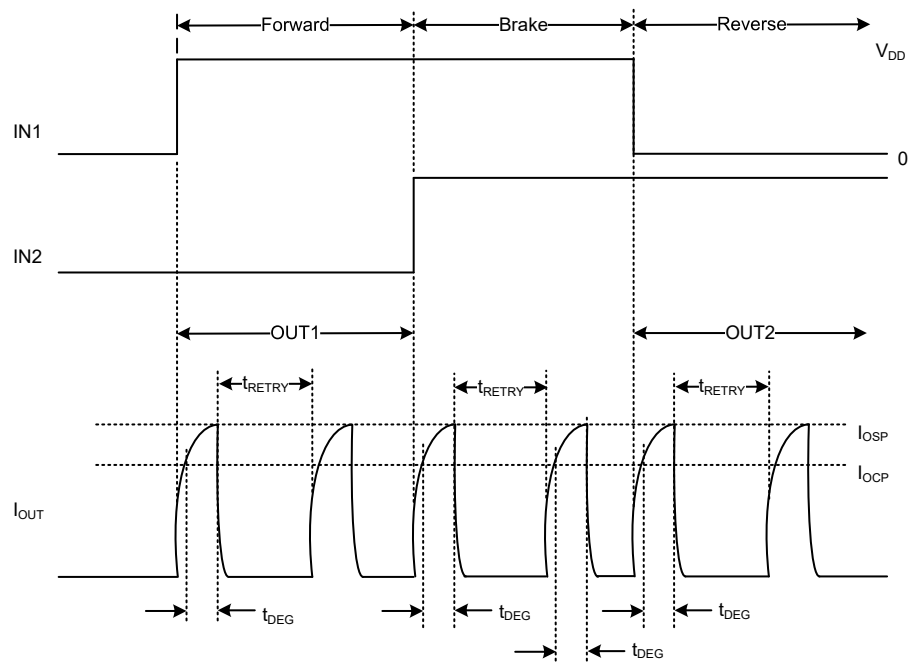
图 5. 重试响应
