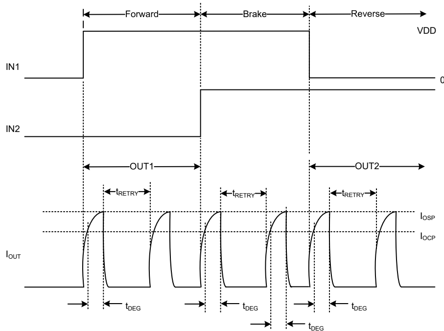
图 6. 重试机制
