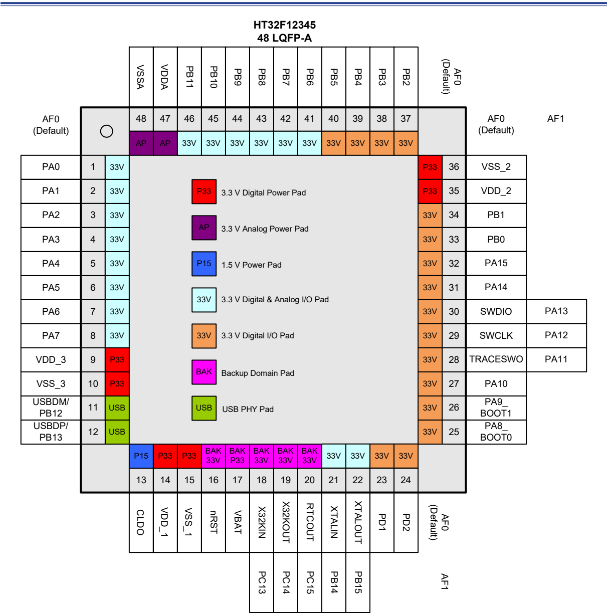
图 5. 48-pin LQFP 引脚图
