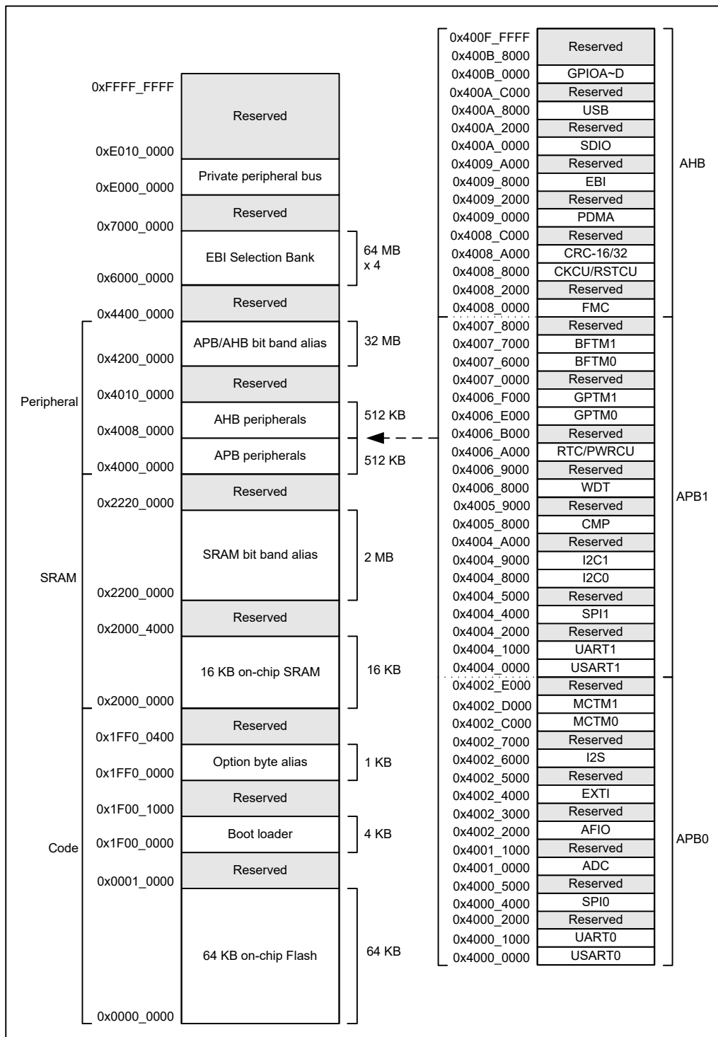
图 2. 存储器映射
