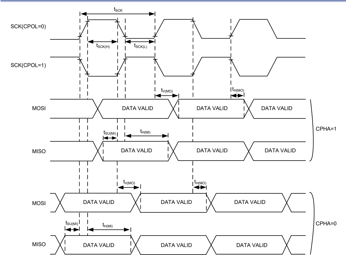
图 9. SPI 时序图 – SPI 主机模式
