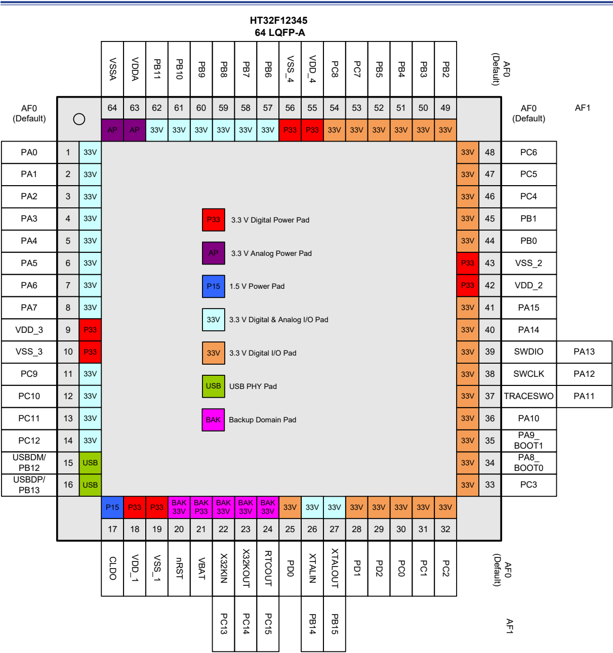
图 6. 64-pin LQFP 引脚图
