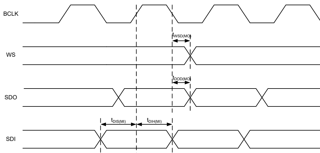
图 11. I²S 主机模式时序图
