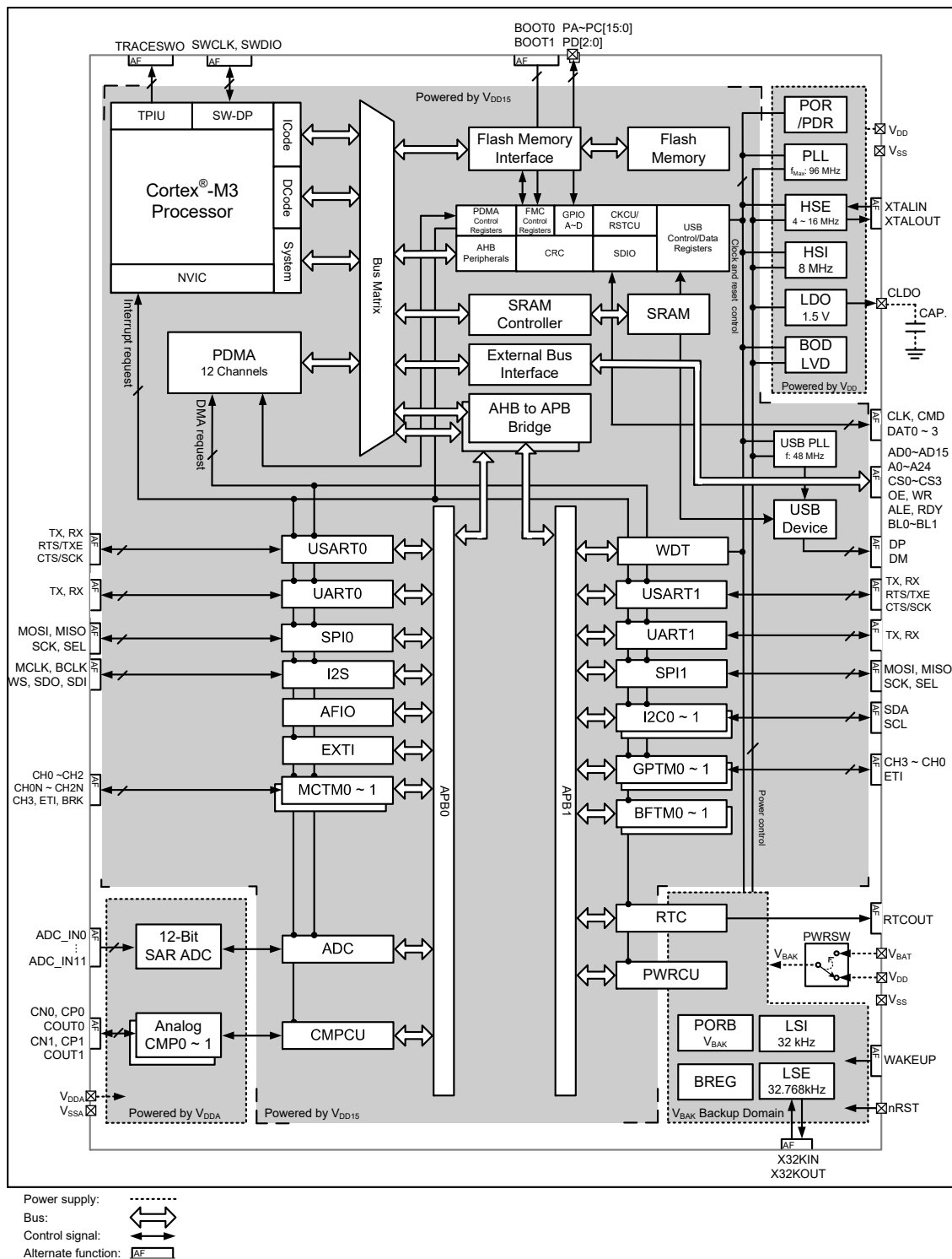
图 1. 方框图
