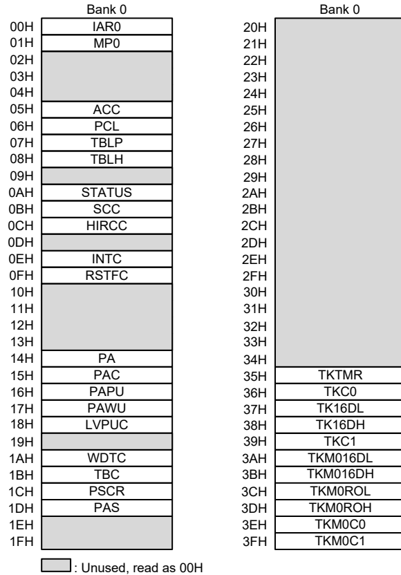
特殊功能数据存储结构
