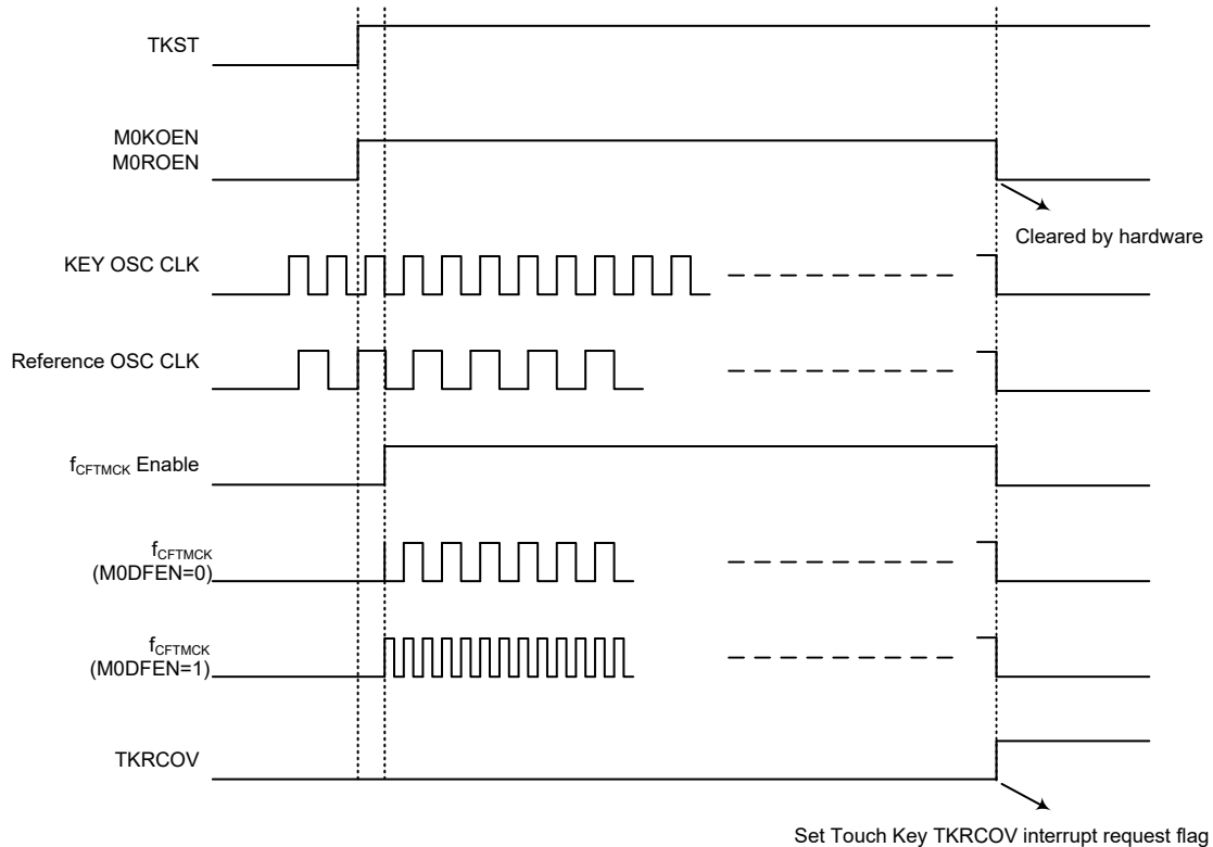
触控按键扫描模式时序图
