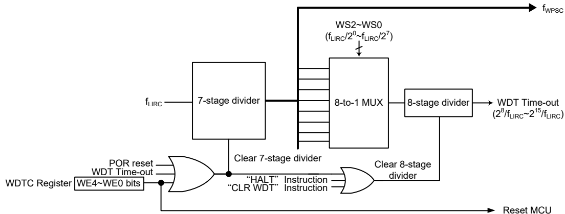
看门狗定时器
