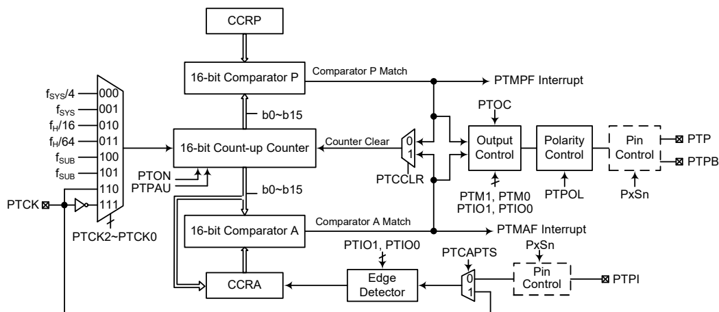
16-bit 周期型 TM 方框图
